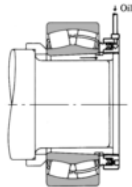
Ausbau unter Verwendung einer Hydraulikmutter
