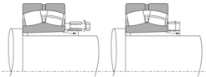
Ausbau der Abziehhülse mit Abziehmutter und Druckschrauben
