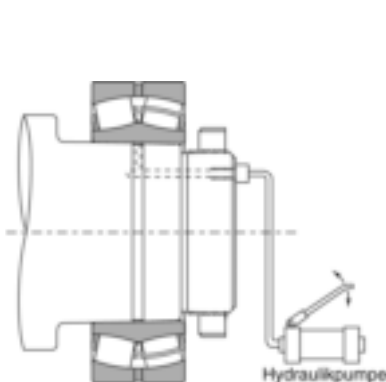
Ausbau unter Öleinspritzung
